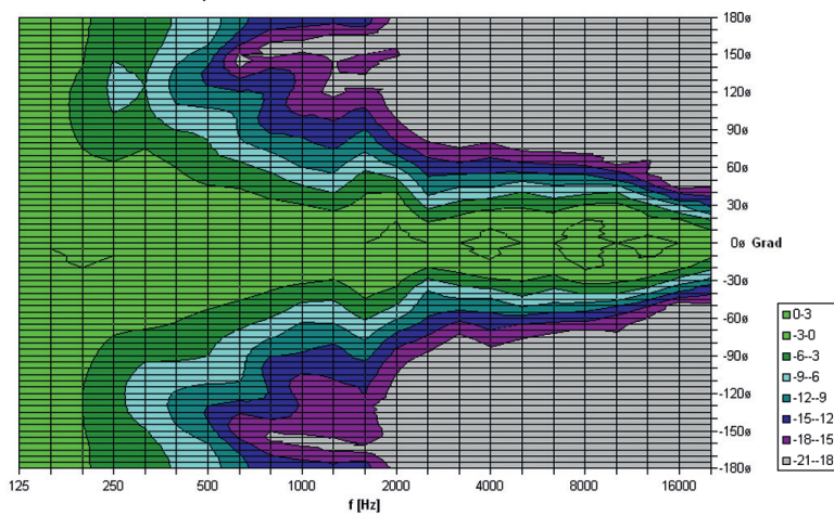
F 10 A vert. Direktivität Plot
